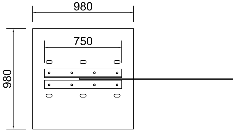
PLACA VIENTOS TIPO1- SIMPLE (conjun.enterrado)
